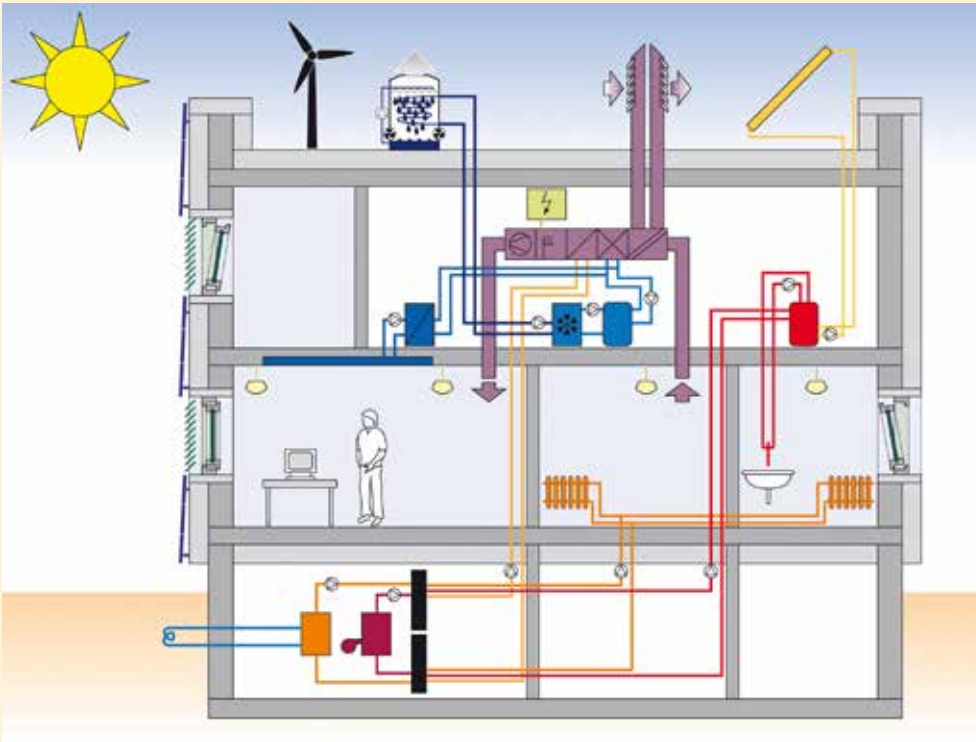
Schematische Darstellung des Bilanzumfangs der DIN V 18599
