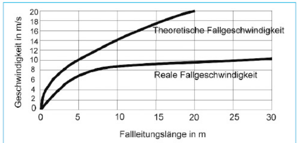
Bild 4 Theoretische und reale Fallgeschwindigkeit in Fallleitungen
