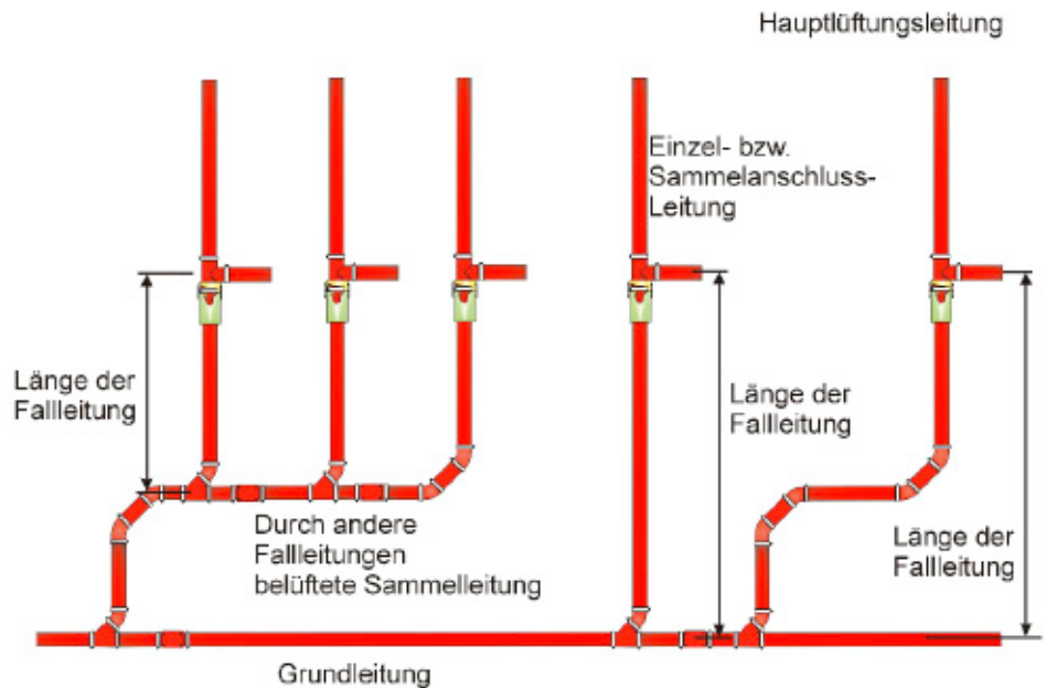
Bild 1 „Bezüge für die Ermittlung der Falleitungslänge“ aus DIN-Kommentar
