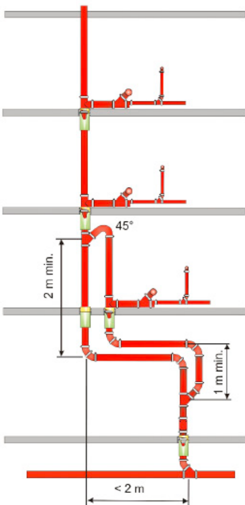
Bild 11 Falleitungsverziehung < 2 m mit Umgehungsleitung (Bild 8 aus DIN 1986-100)
