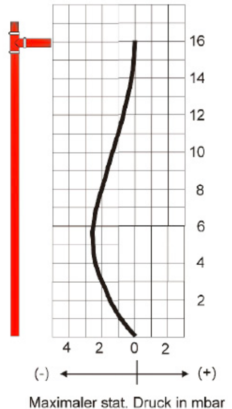
Bild 2 Druckverlauf in einer Schmutzwasser-Falleitung
