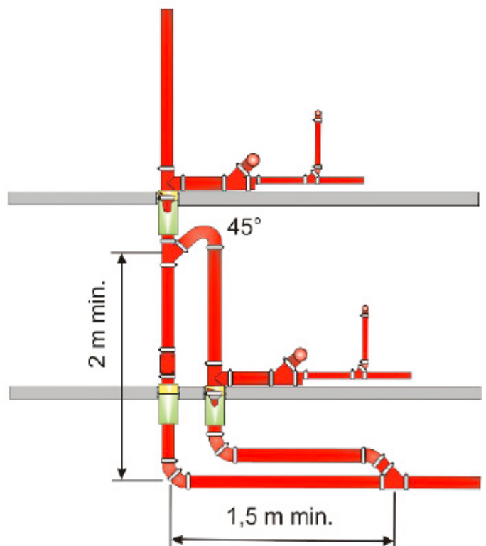
Bild 12 Falleitungsverziehung \geq 2 m mit Umgehungsleitung oder Umgehungsleitung für den Übergang einer Falleitung in die Sammel- oder Grundleitung (Bild 11 aus DIN 1986-100)
