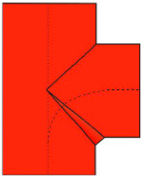
Bild 3 87° Anschluss-Abzweige sind strömungstechnisch ungünstiger als Abzweige mit 45° Einlaufwinkel
