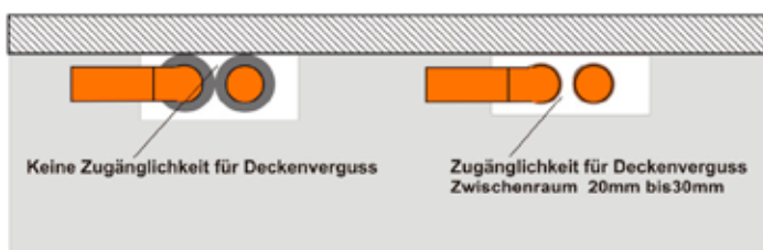
Bild 2 Problemzonen bei Null-Abstand.
