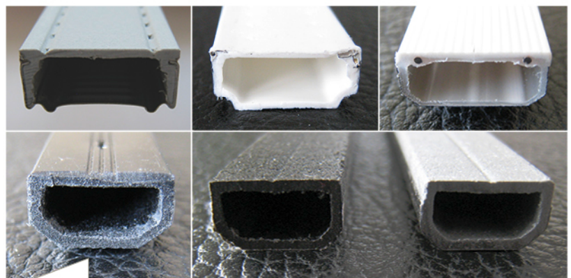
Kunststoff-Spacer Typ I (oben v. l.): Chromatech Ultra, TGI Spacer M, Thermix TX.N plus Kunststoff-Spacer Typ II (unten v. l.): Thermobar, Swisspacer Advance / Ultimate
